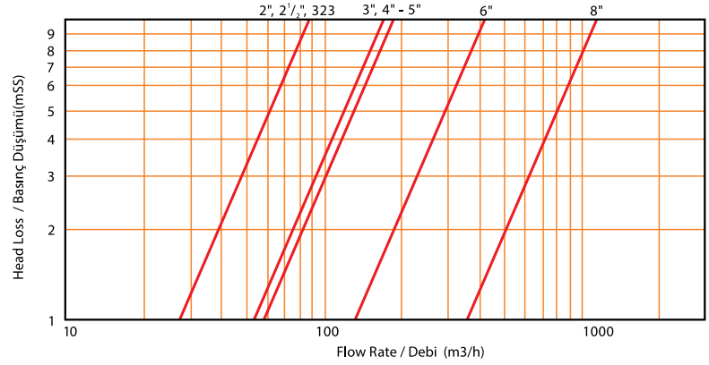
Head Loss Chart / Basınç Düşümü Tablosu
