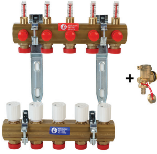
R553F Debi Göstergeli Pirinç Kollektör Brass Manifold With Dynamic Flow Balancing
