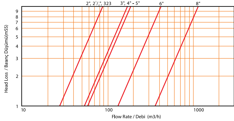
Head Loss Chart / Basınç Düşümü Tablosu
